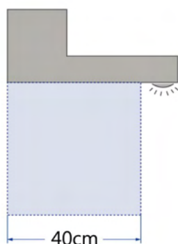
市售T型排油煙機
